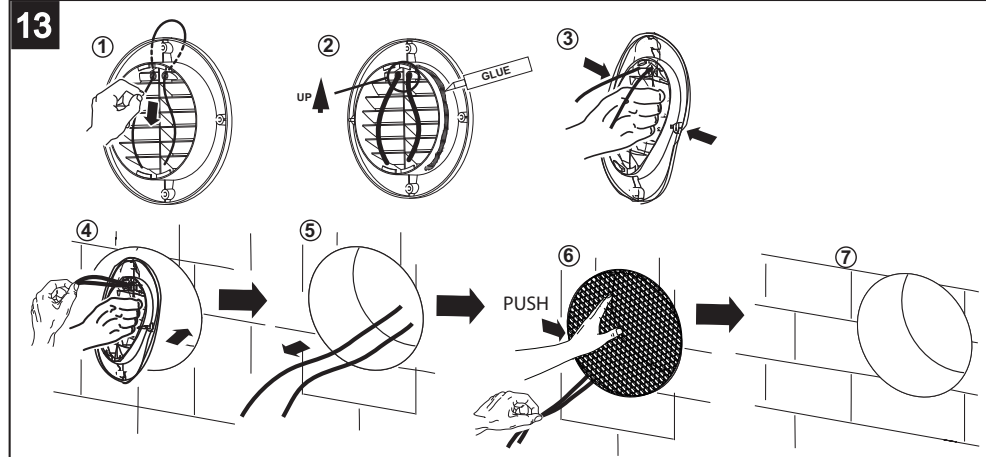
VORT HRW 40 MONO EVO - 由内部安装格栅
