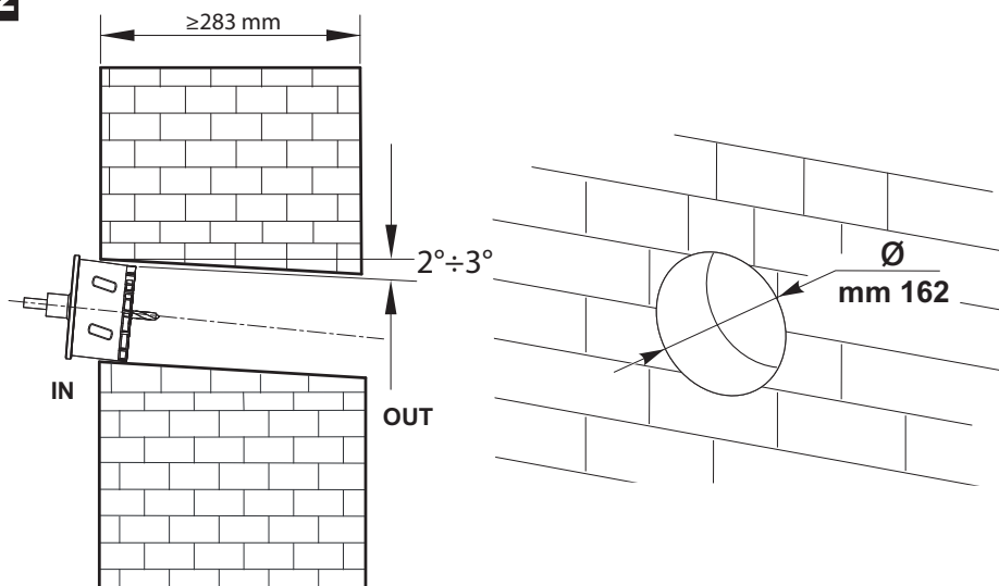
VORT HRW 40 MONO EVO - MONTAGE DES GITTERS VON INNEN
