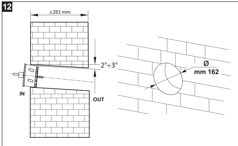
VORT HRW 40 MONO EVO - RÁCS BESZERELÉSE BELÜLRŐL
