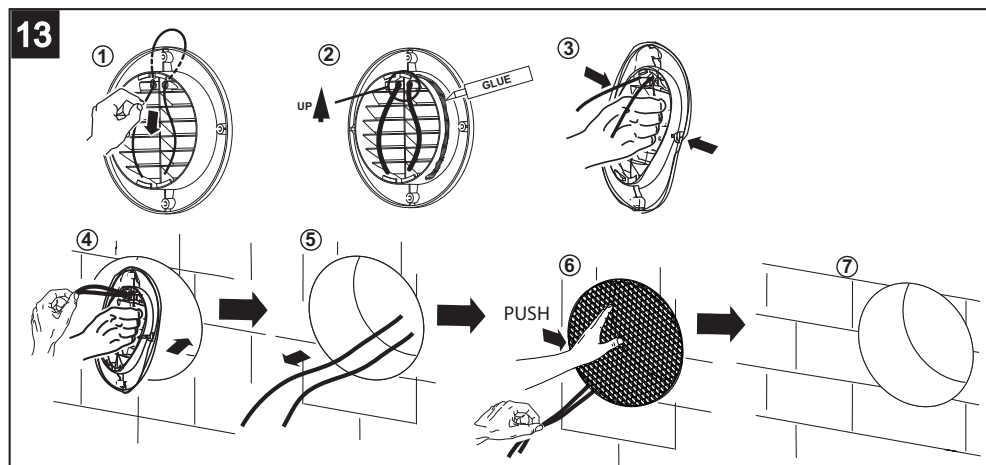
VORT HRW 40 MONO EVO - RÁCS BESZERELÉSE BELÜLRŐL
