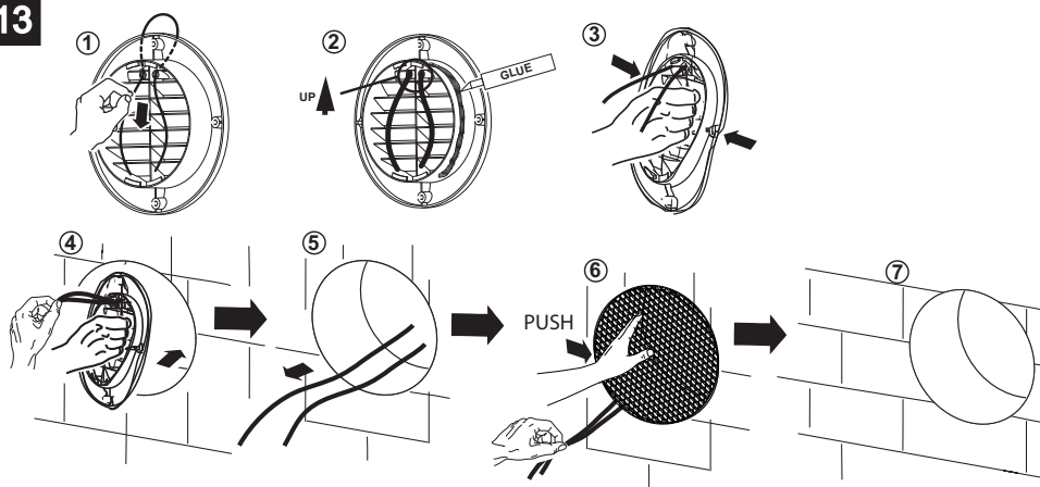
VORT HRW 40 MONO EVO - MONTAGGIO GRIGLIA DALL'INTERNO
