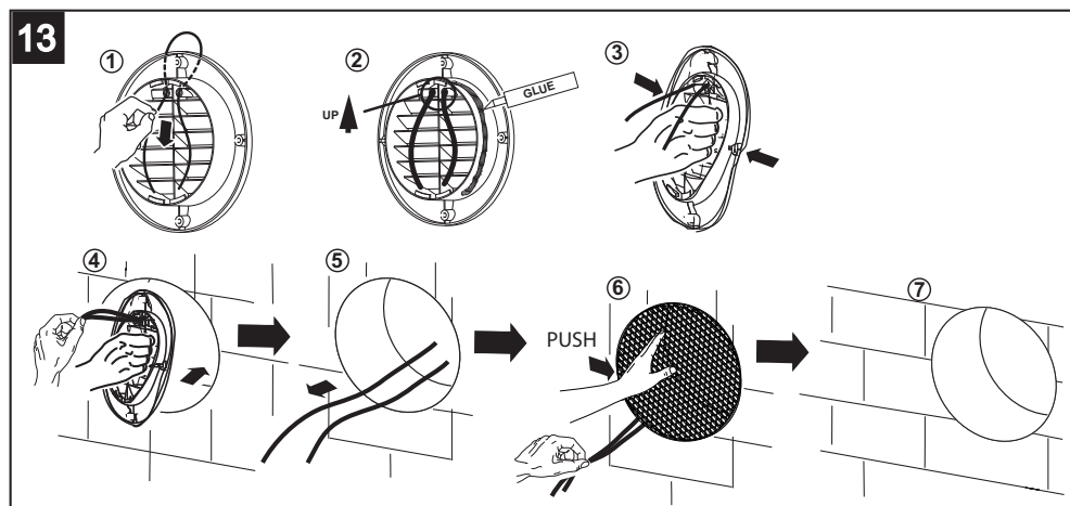
VORT HRW 40 MONO EVO - MONTAJE REJILLA DESDE EL INTERIOR
