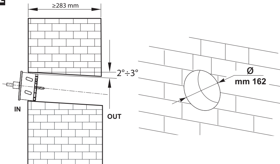
VORT HRW 40 MONO EVO - MONTAGGIO GRIGLIA DALL'INTERNO
