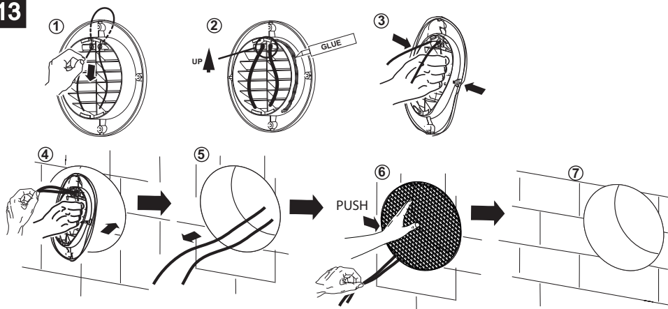
VORT HRW 40 MONO EVO - MONTAGE DES GITTERS VON INNEN
